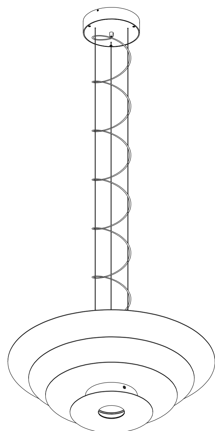
PL312 D550xH1200(mm) SMD-18W+COB-9W
