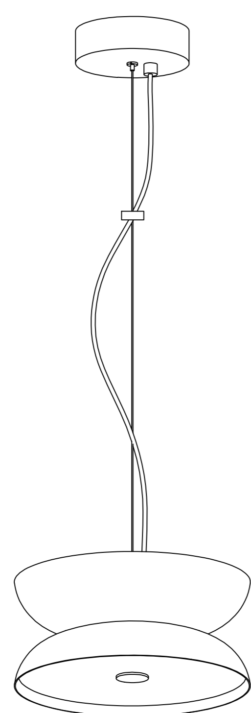
PL335 D220xH2000(mm) LED-2x10W
